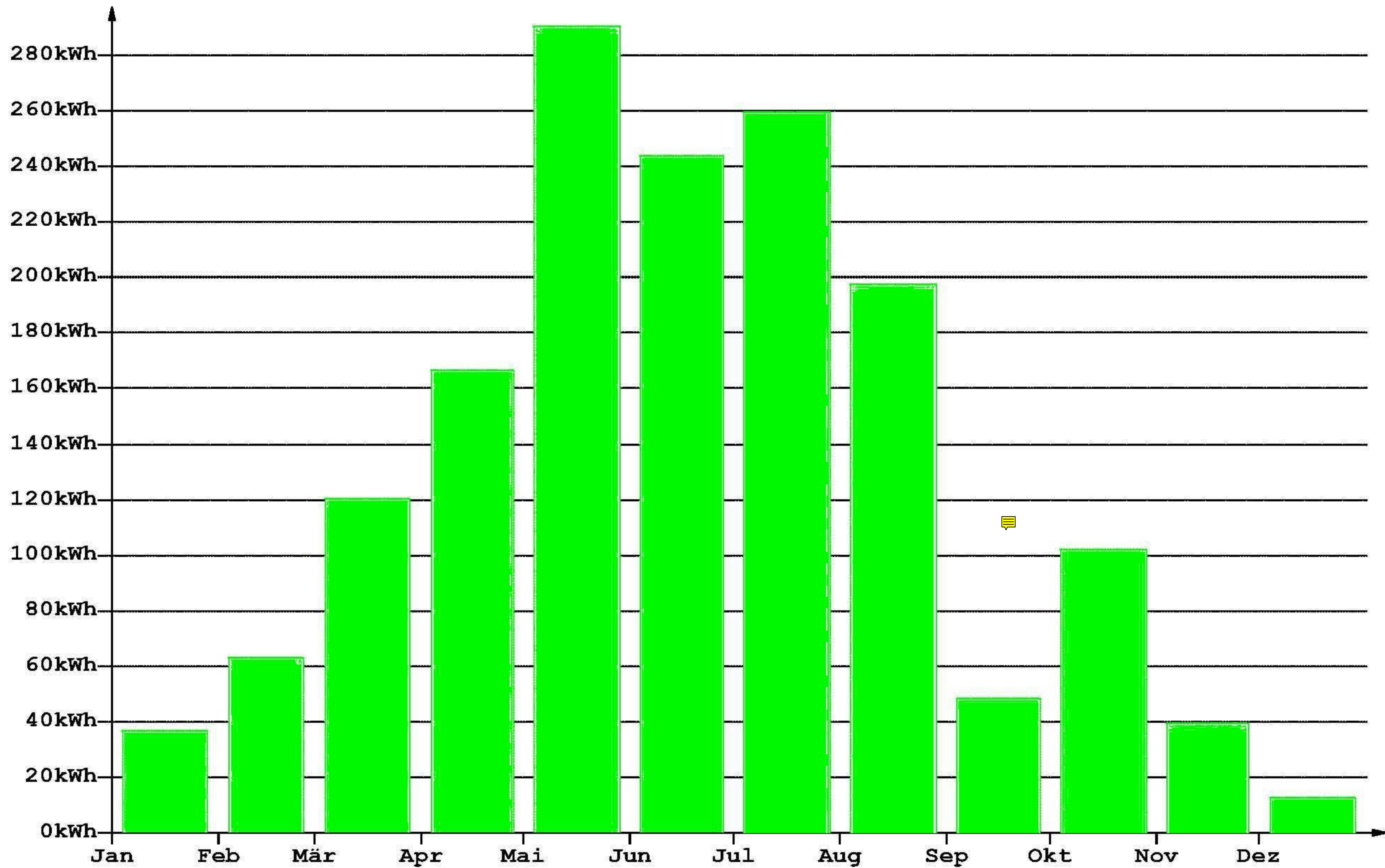
eingespeiste Energie im Jahr 2001
