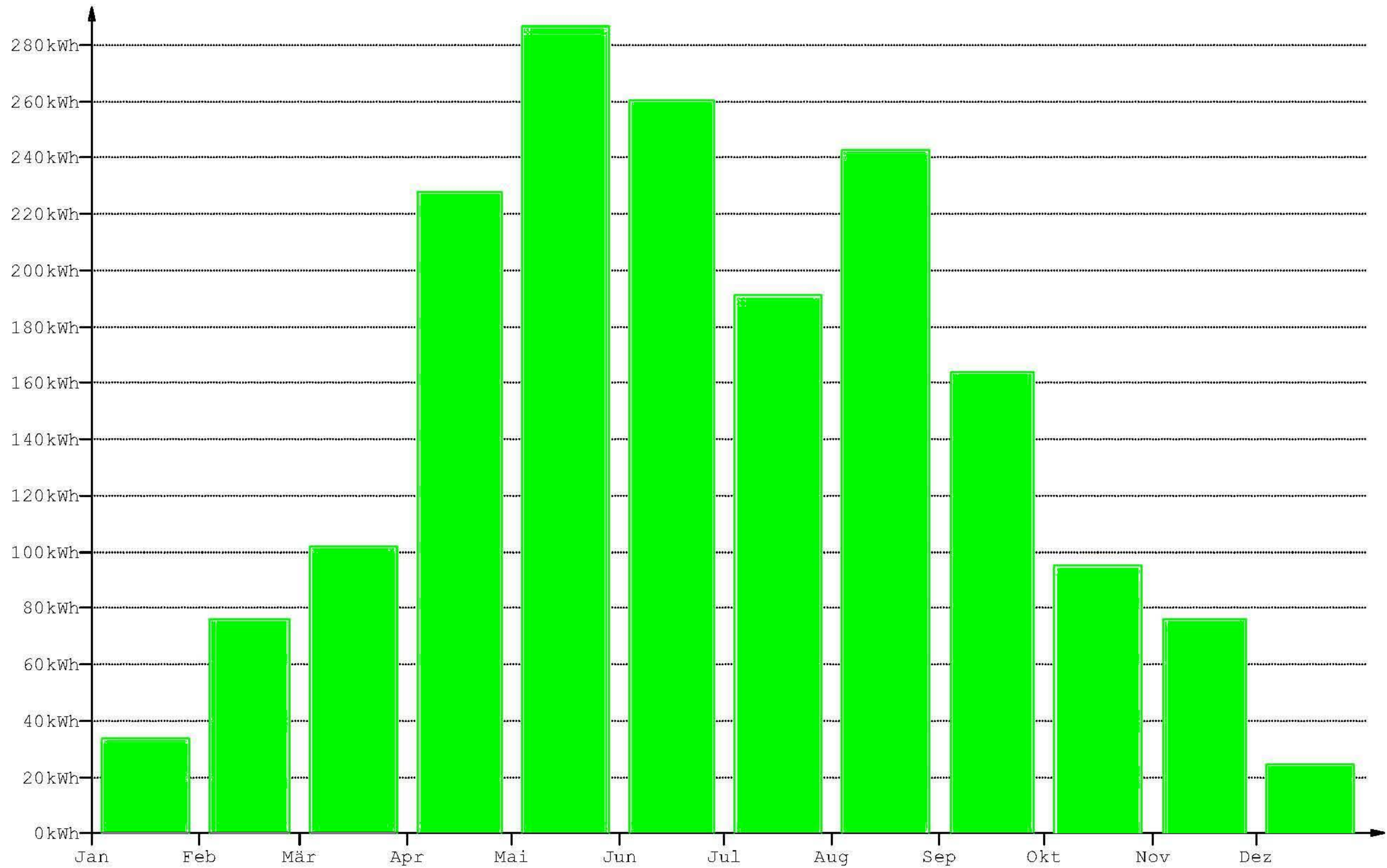
eingespeiste Energie im Jahr 2000
