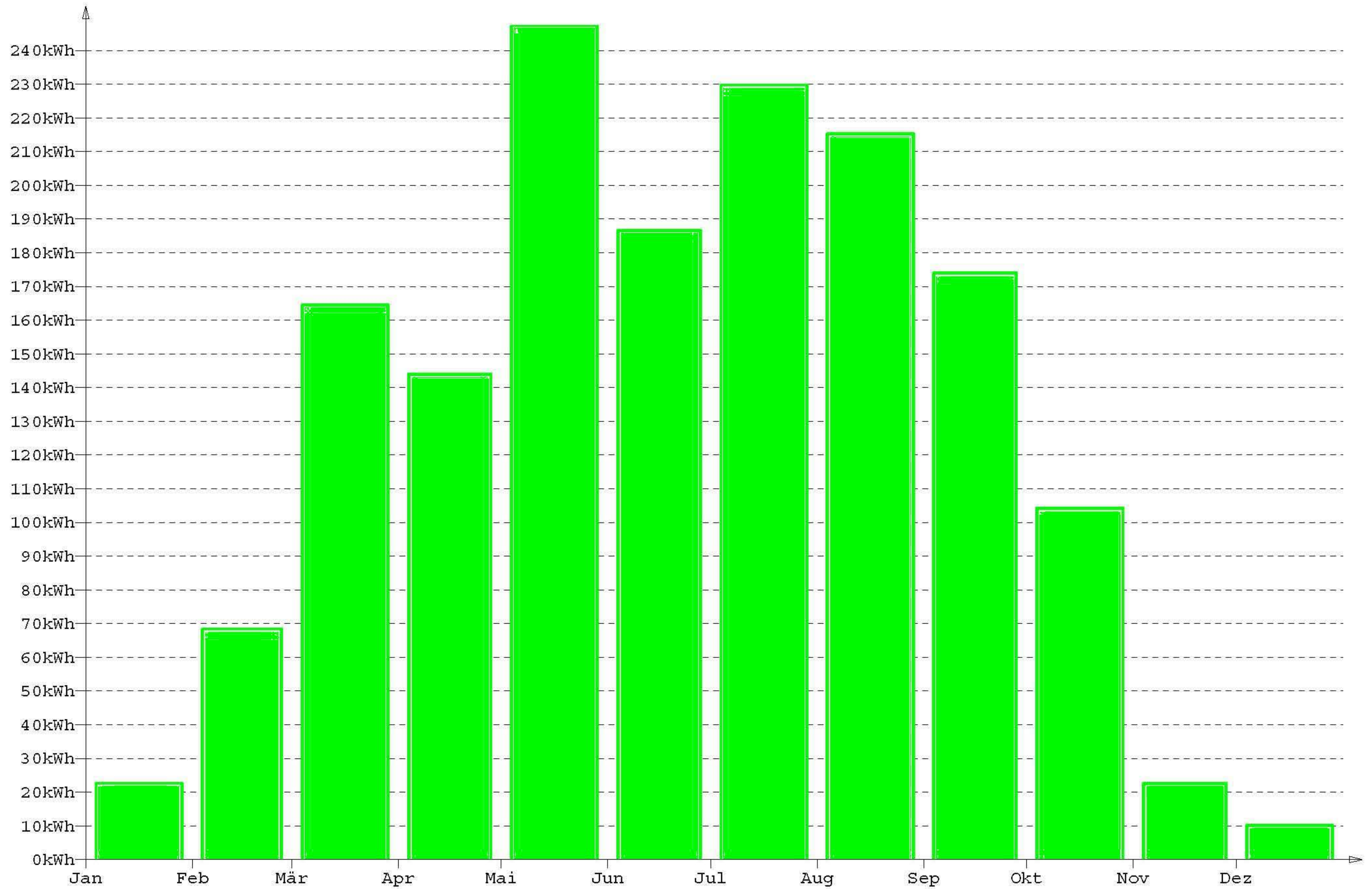
eingespeiste Energie im Jahr 2012
