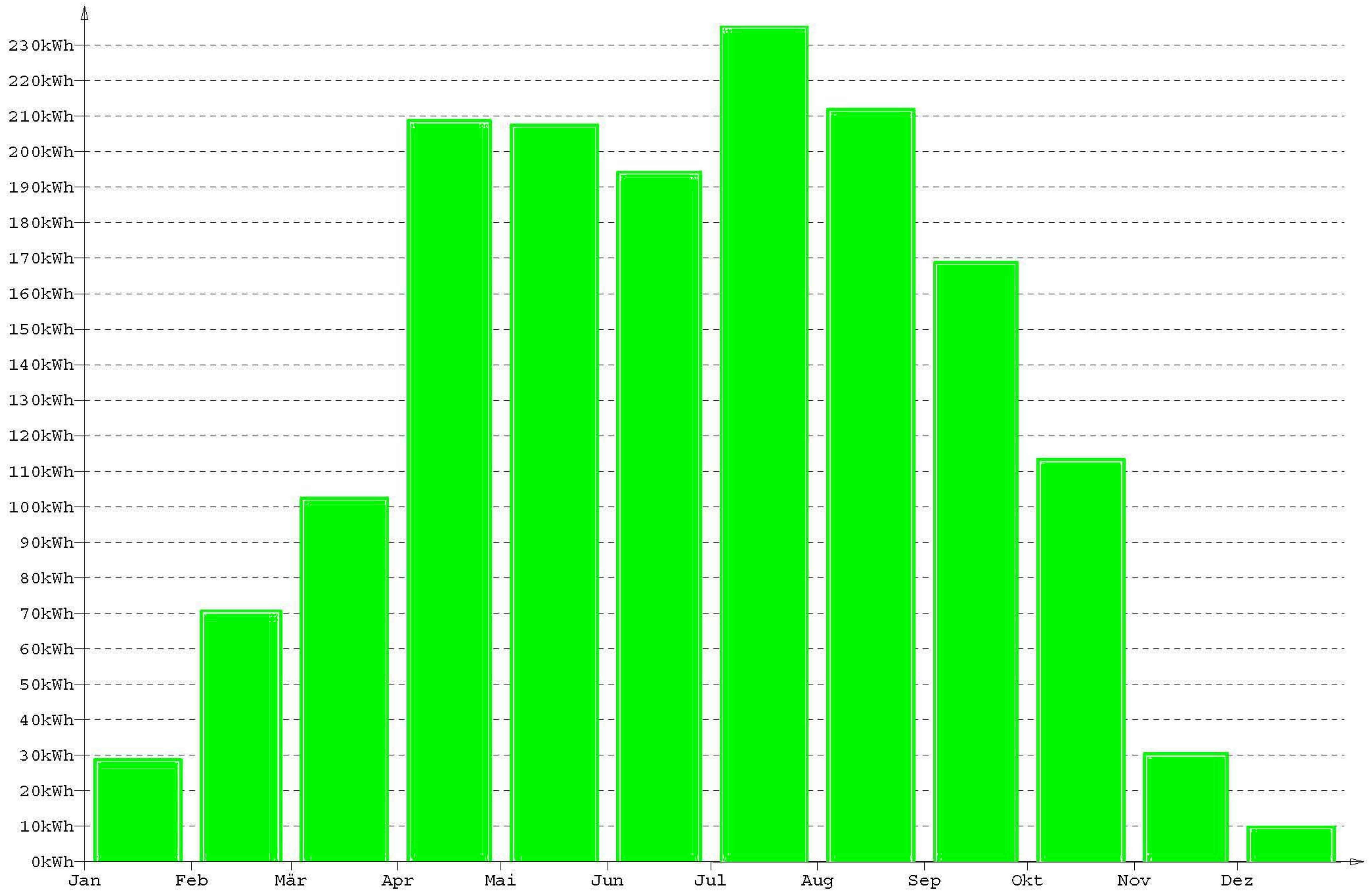
eingespeiste Energie im Jahr 2004
