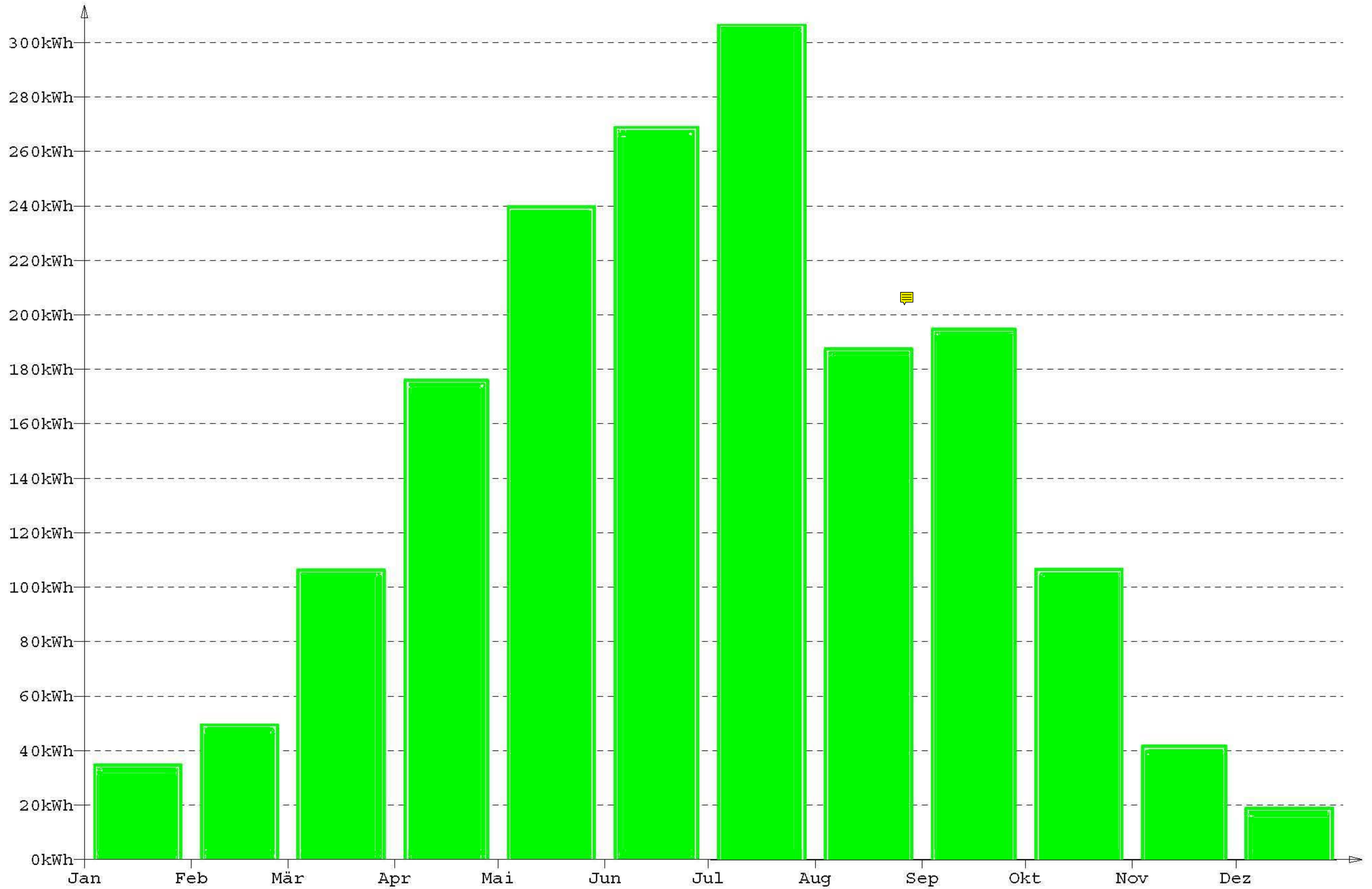
eingespeiste Energie im Jahr 2006
