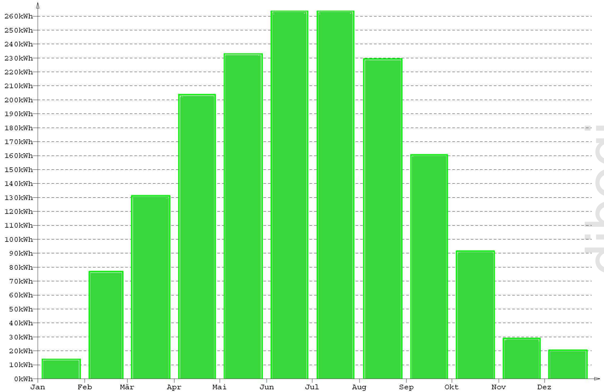
eingespeiste Energie im Jahr 2015
