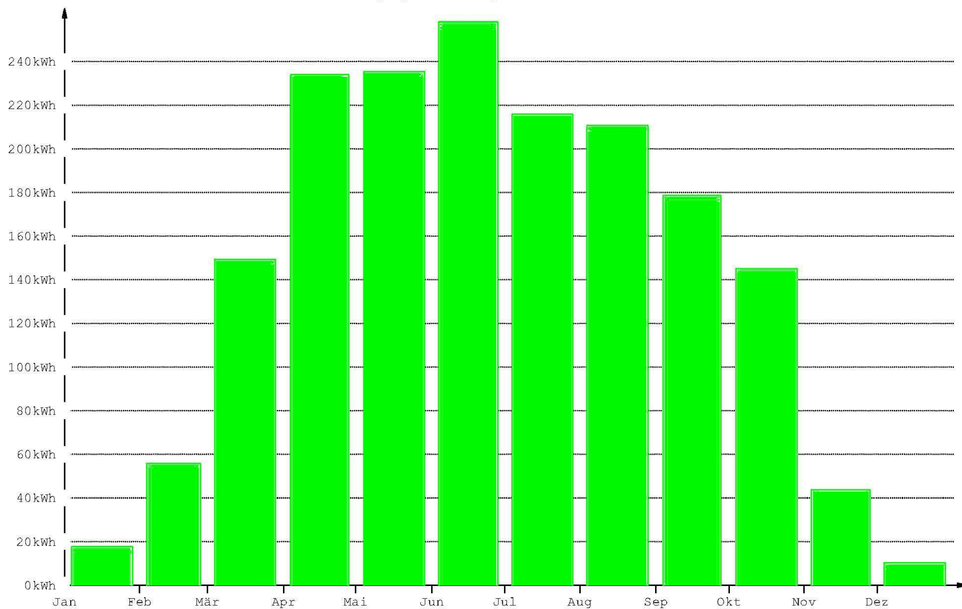
eingespeiste Energie im Jahr 2005
