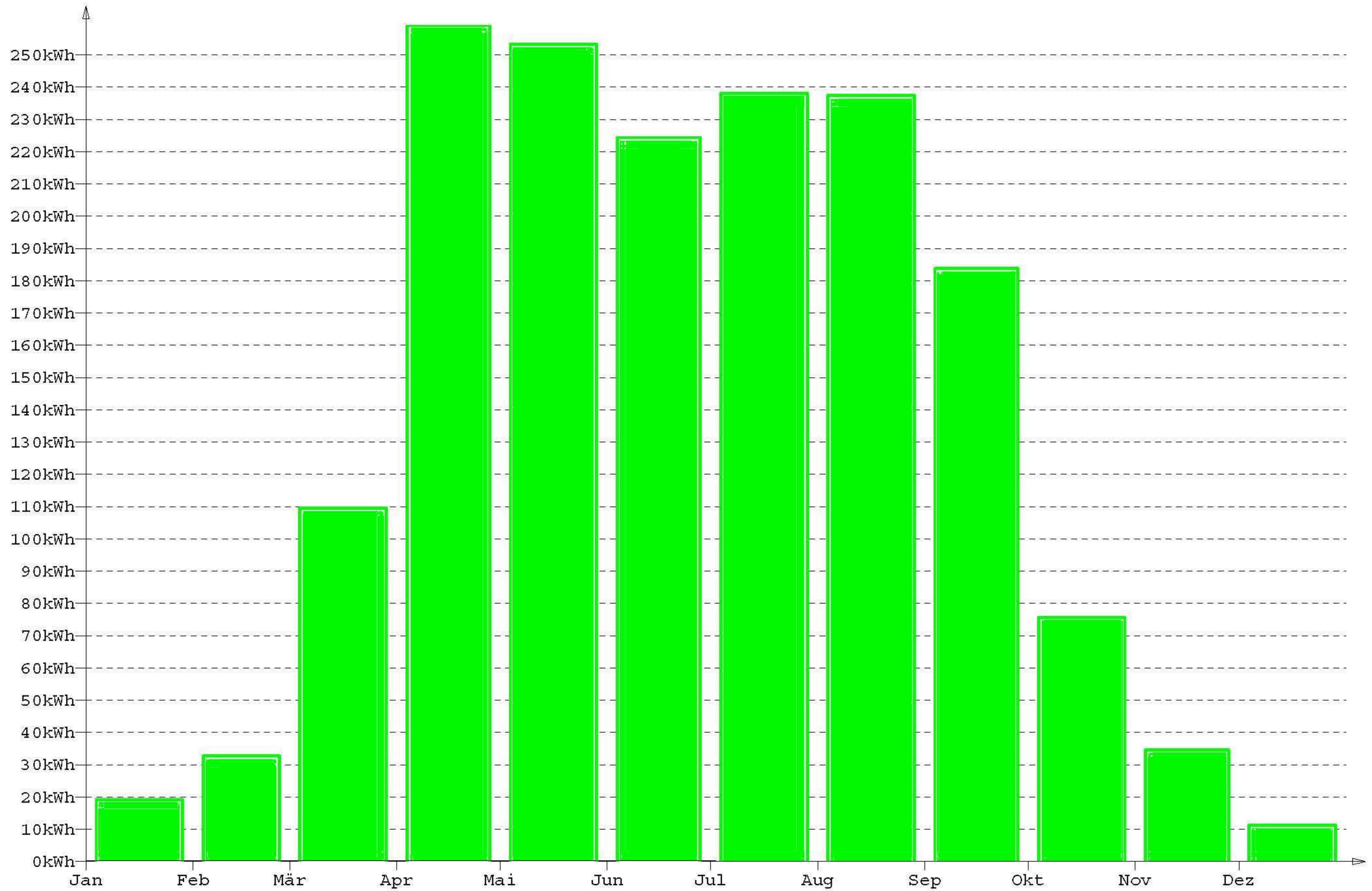
eingespeiste Energie im Jahr 2009
