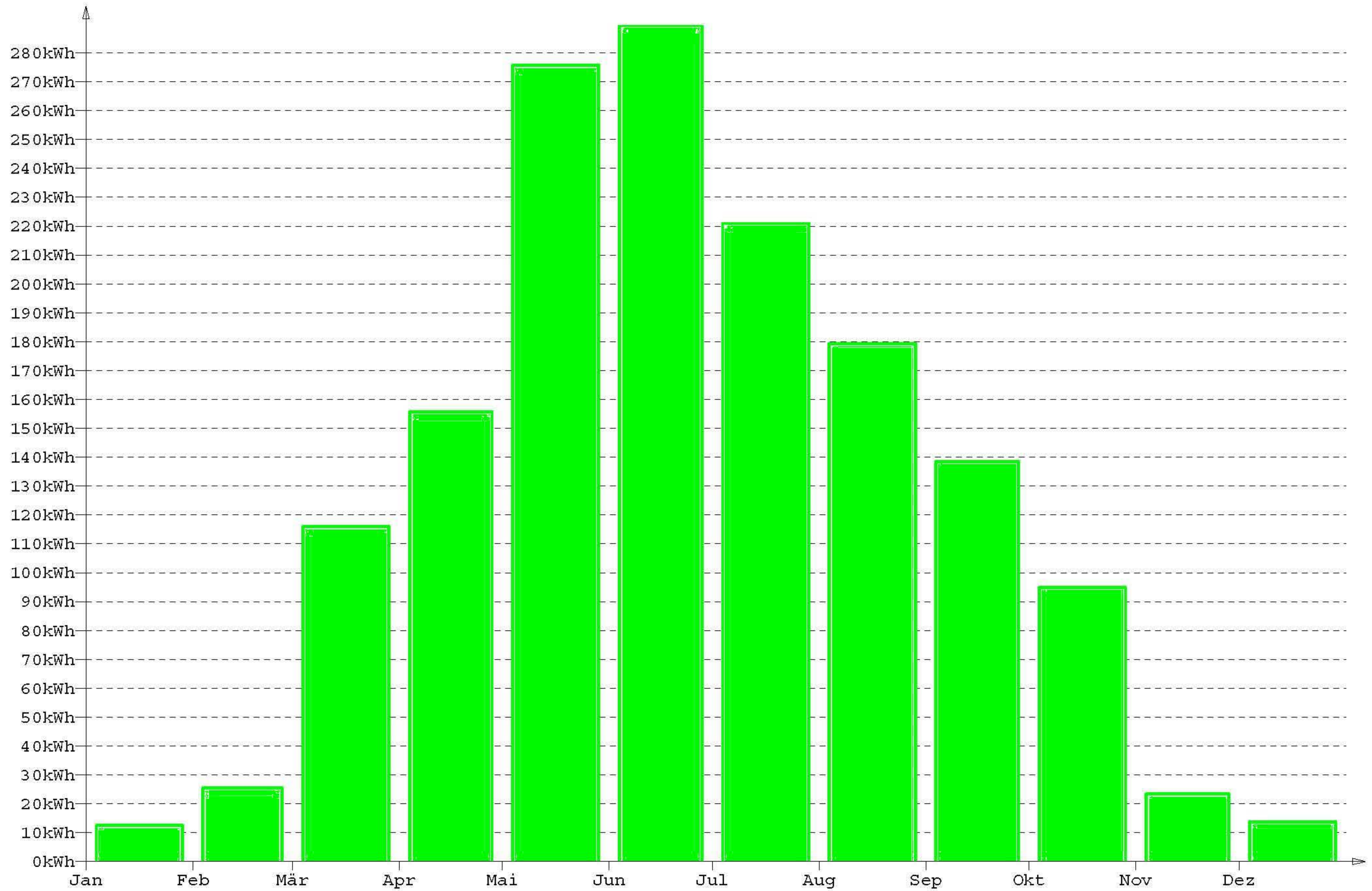
eingespeiste Energie im Jahr 2008
