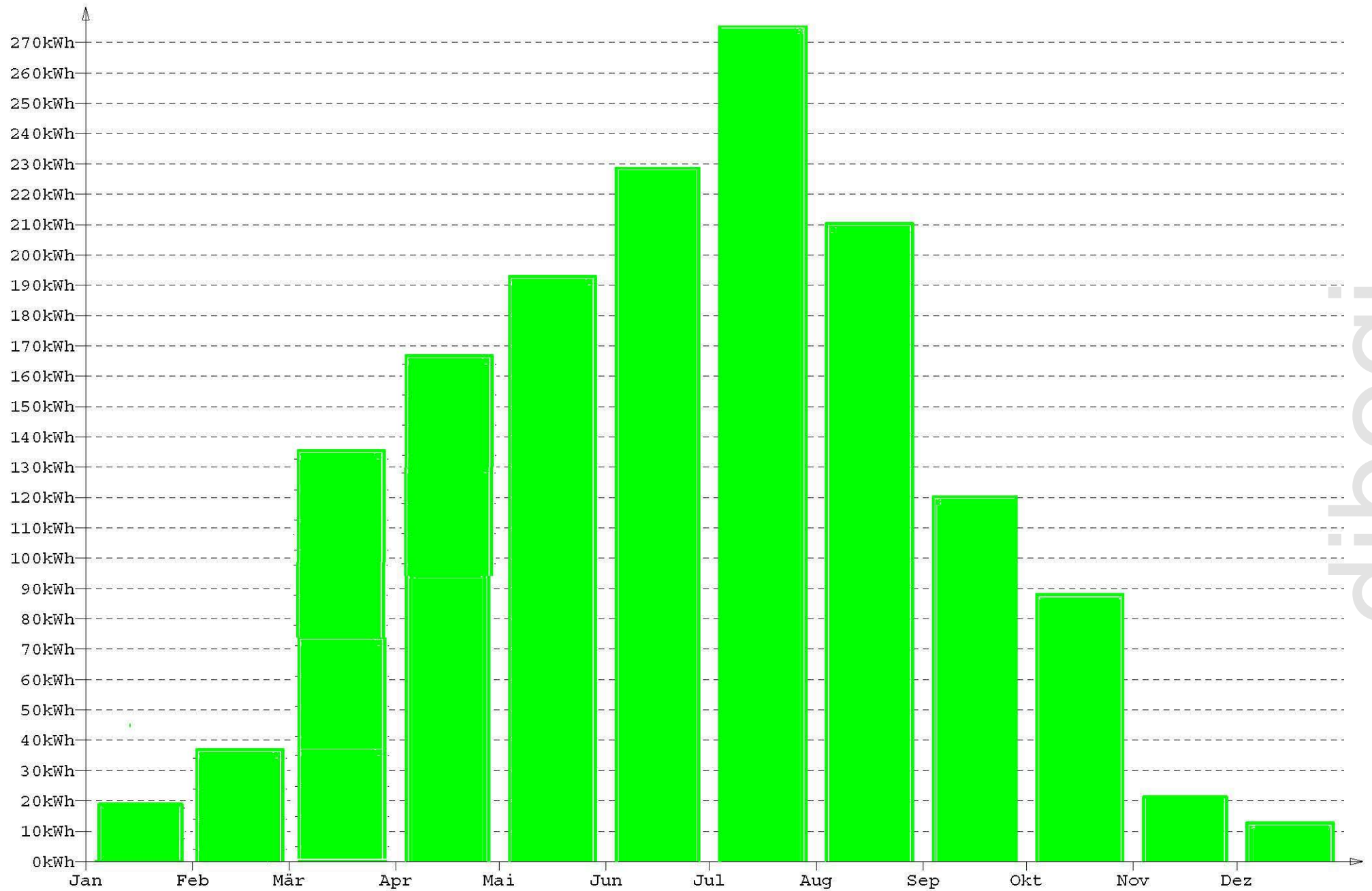
eingespeiste Energie im Jahr 2013
