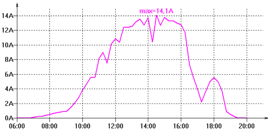
Solarzellenstrom
