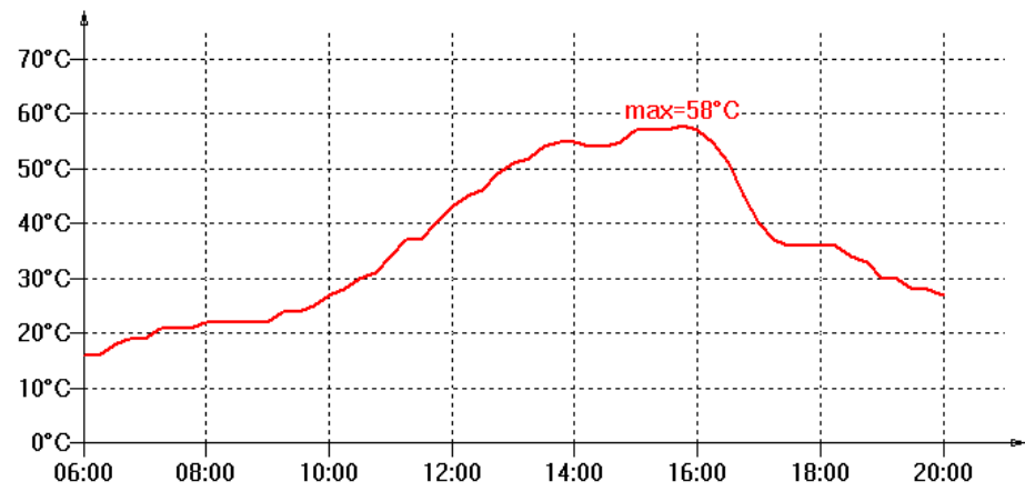
Wechselrichter-Temperatur
